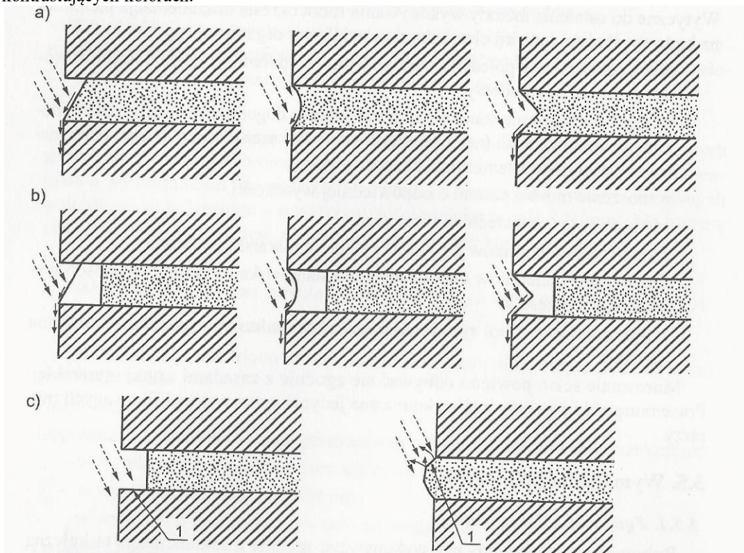
a – spoinowanie prawidłowe, b – spoinowanie nie zalecane ze względów wytrzymałościowych, c – spoinowanie nieprawidłowe z uwagi na możliwość zawilgocenia muru 1 – miejsce zawilgocenia
