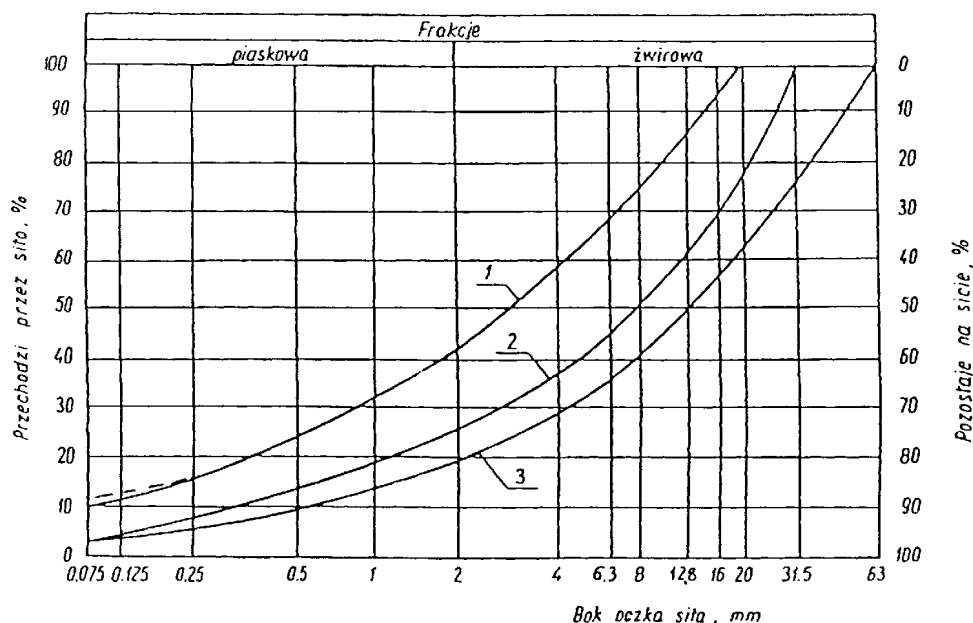
Rysunek 1. Pole dobrego uziarnienia kruszyw przeznaczonych na podbudowy (nawierzchnię) wykonywane metodą stabilizacji mechanicznej
