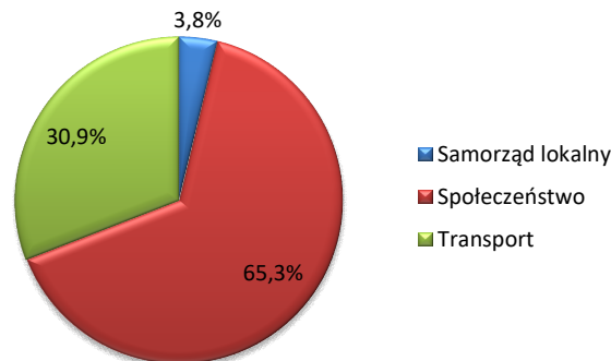
Ryc. 21 Procentowy udział emisji CO 2 w poszczególnych sektorach w 2017 r.
