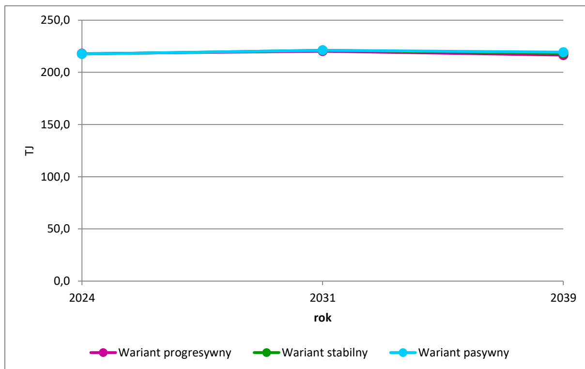
Rysunek 28. Prognozowana zmiana zużycia ciepła do roku 2039.
