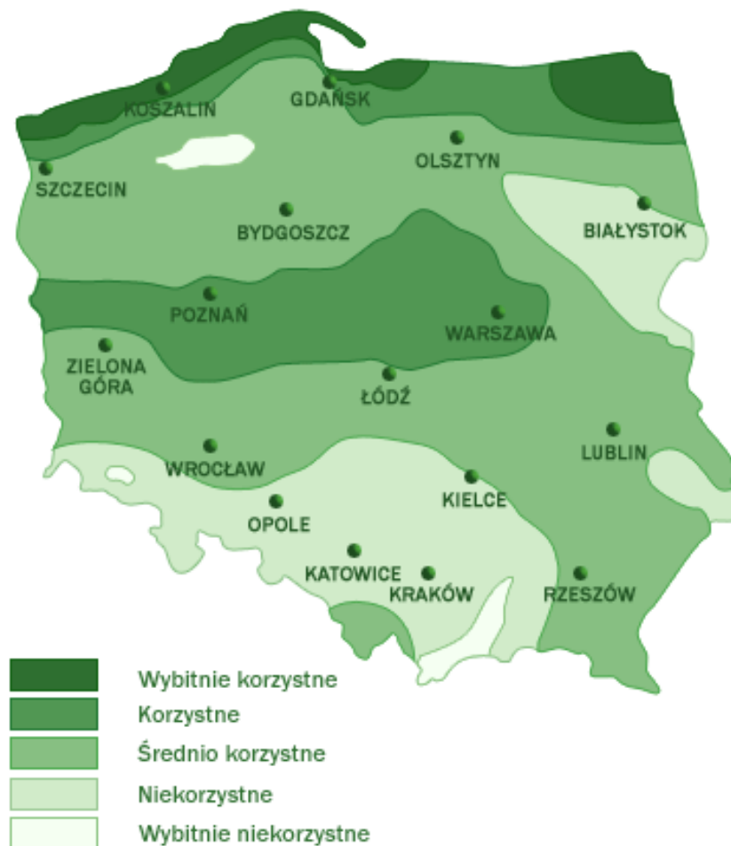
Rysunek 24. Strefy energetyczne warunków wiatrowych. źródło: IMGW
