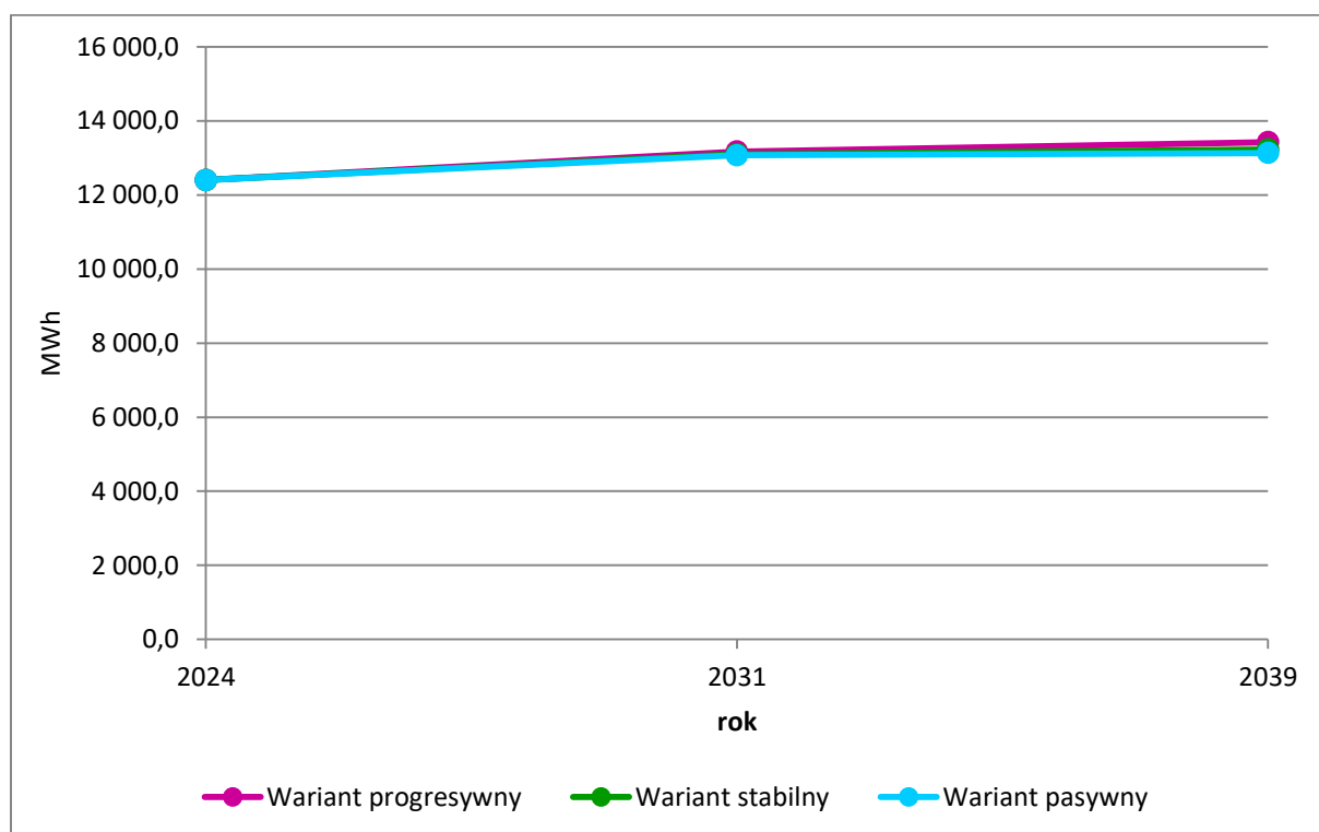
Rysunek 30. Prognozowana zmiana rocznego zużycia energii elektrycznej do roku 2039.
