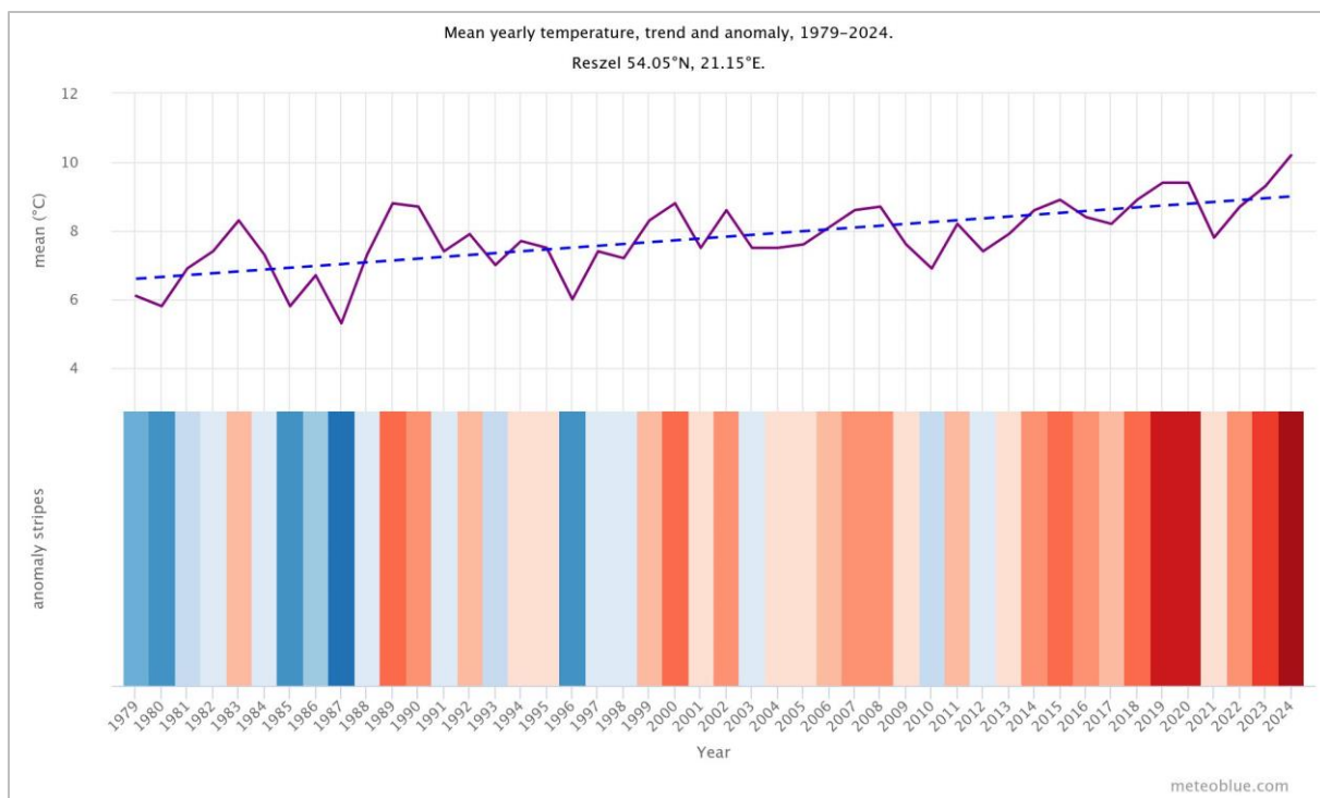
Rysunek 21. Roczna zmiana temperatury w Reszlu. źródło: www.meteoblue.com
