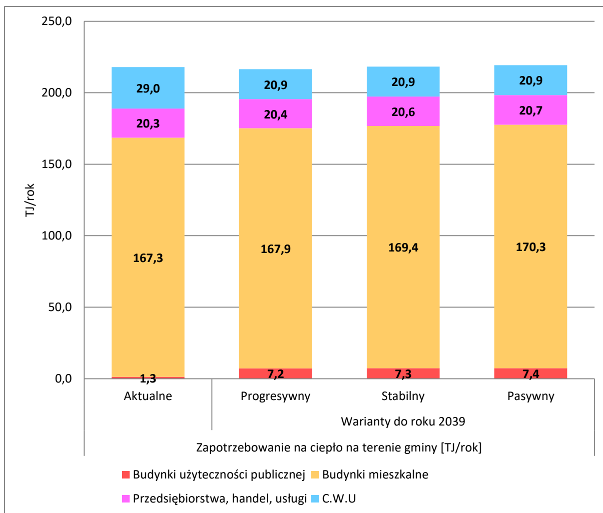
Rysunek 29. Szczegółowy bilans rocznego zapotrzebowania na ciepło na terenie gminy. źródło: opracowanie własne
