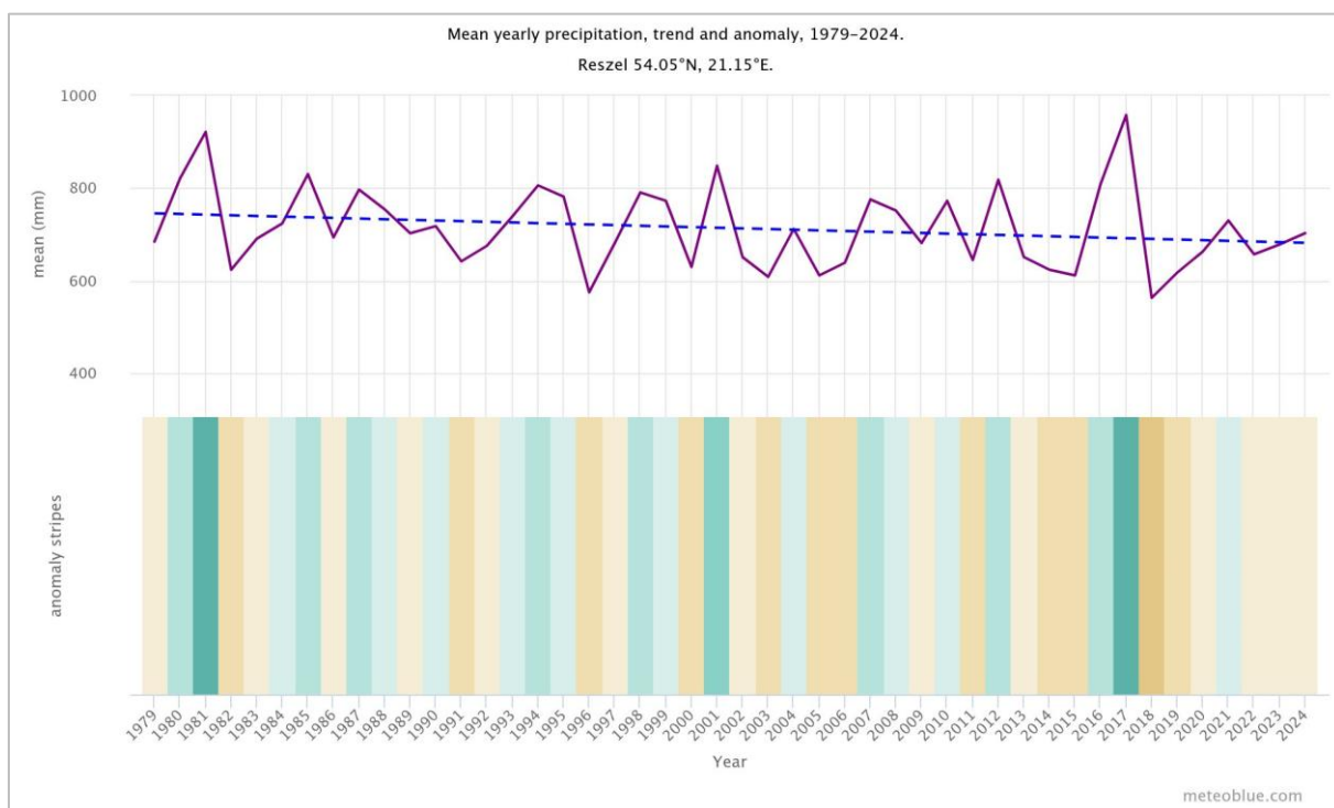
Rysunek 22. Roczna zmiana opadów w Reszlu. źródło: www.meteoblue.com
