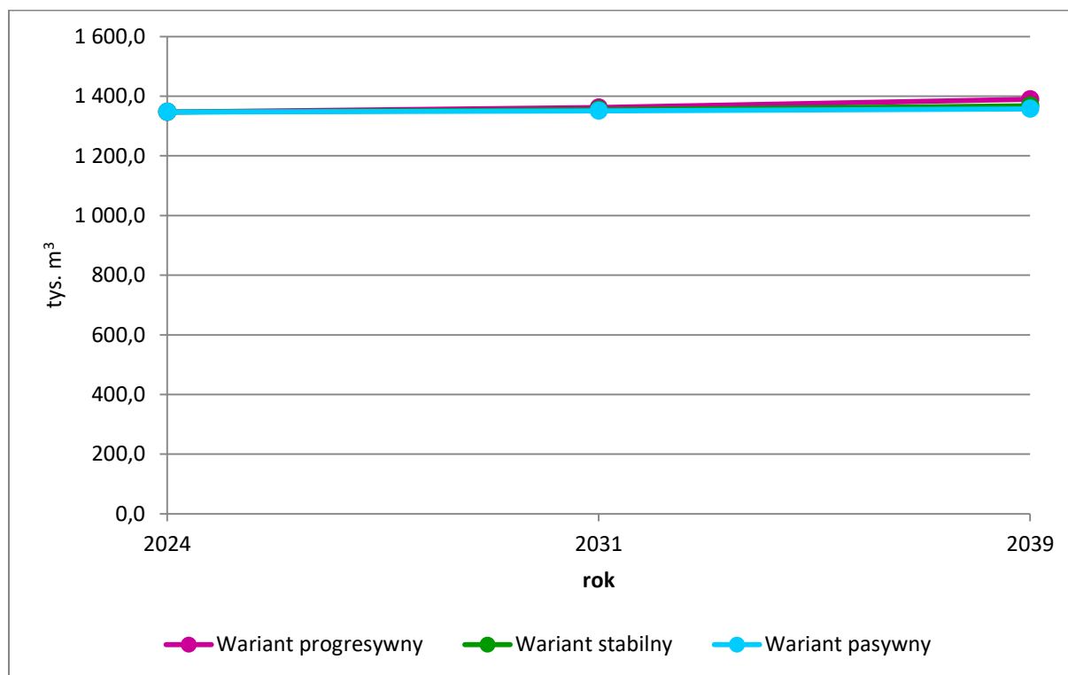
Rysunek 32. Prognozowana zmiana zużycia paliwa gazowego do roku 2039.
