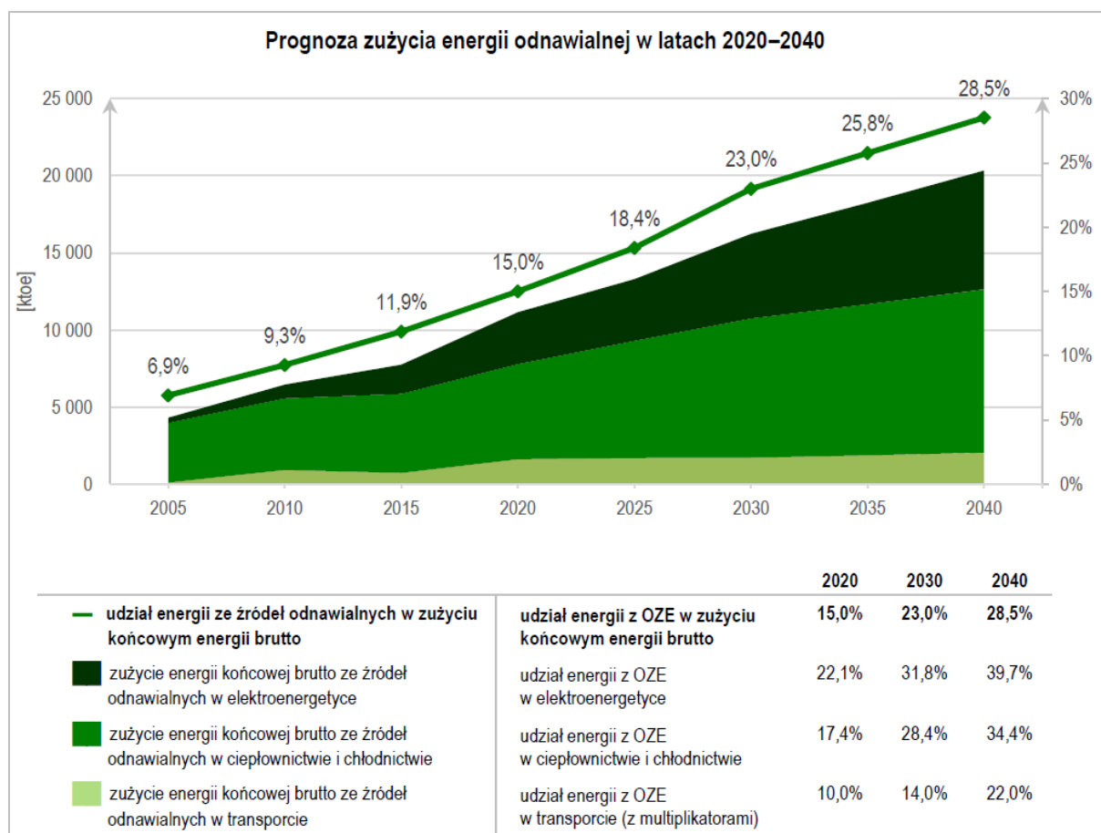
Rysunek 23. Projekcja wzrostu wykorzystania energii odnawialnej w podsektorach, ścieżka wzrostu udziału OZE w końcowym zużyciu energii brutto w perspektywie 2040 r.
