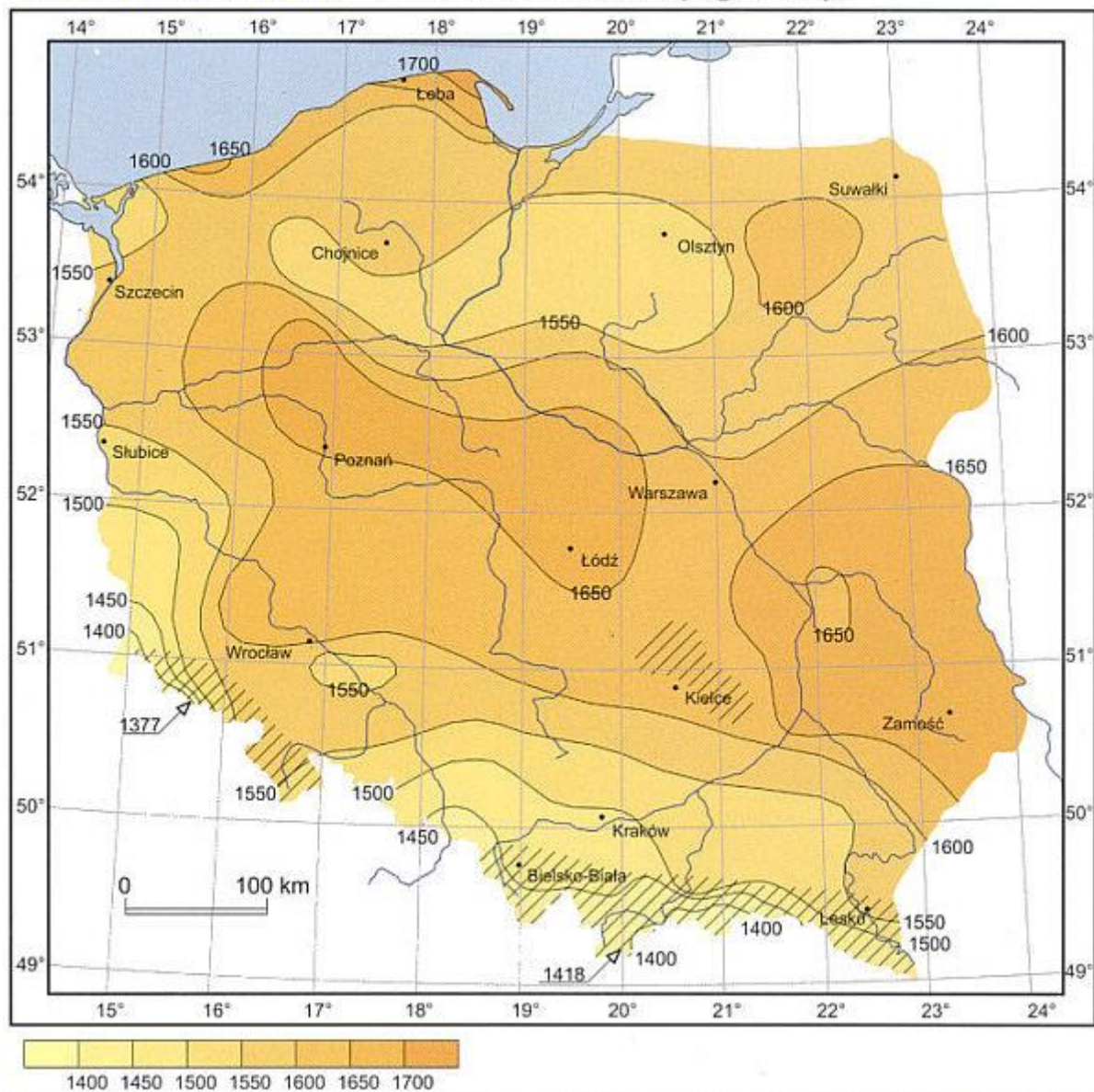
Rysunek 25. Średni czas nasłonecznienia w ciągu roku na terenie Polski [h/rok].
