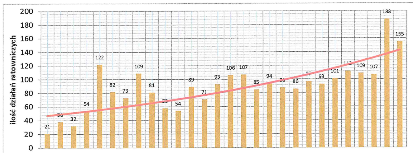
Rys. nr 7. Linia trendu ilości działań ratowniczych jednostek OSP w Gminie Reszel na podstawie ilości działań w latach 1995-2022.
