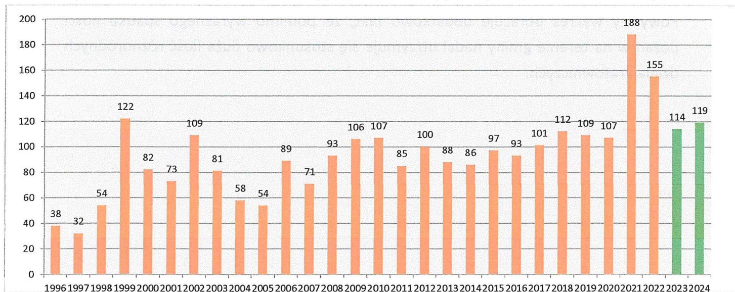
Rys. nr 6. Prognozowana ilość działań ratowniczych w latach 2023, 2024. Badanie przedstawiono na podstawie wyliczeń średniej ruchomej ilości działań w latach 1996-2022.
